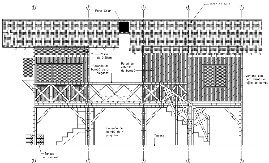
Figura 2. Elevación principal de una vivienda en bambú, Guadua angustifolia .
