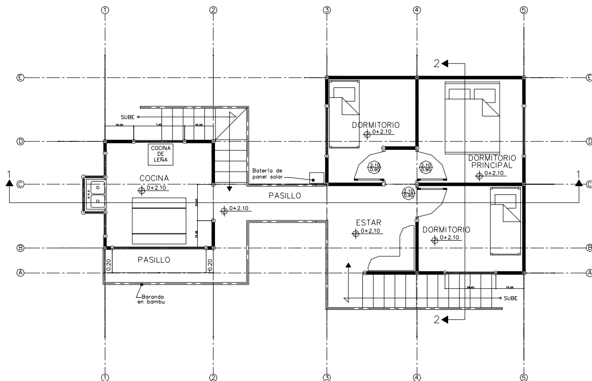
Figura 1. Planta arquitectónica de una vivienda en bambú, Guadua angustifolia .
