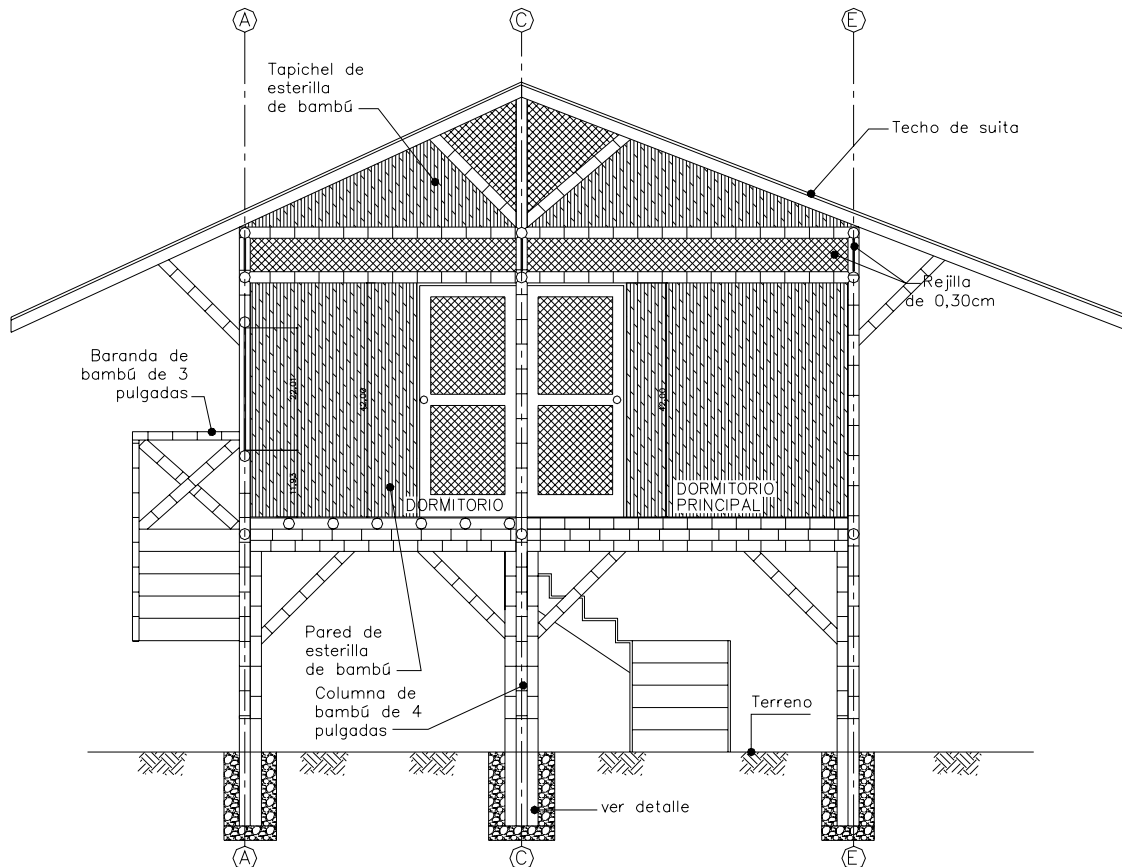
Figura 3. Corte 2 - 2 de una vivienda en bambú, Guadua angustifolia .
